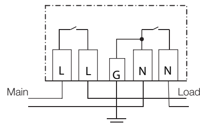
Diagram Koneksi
